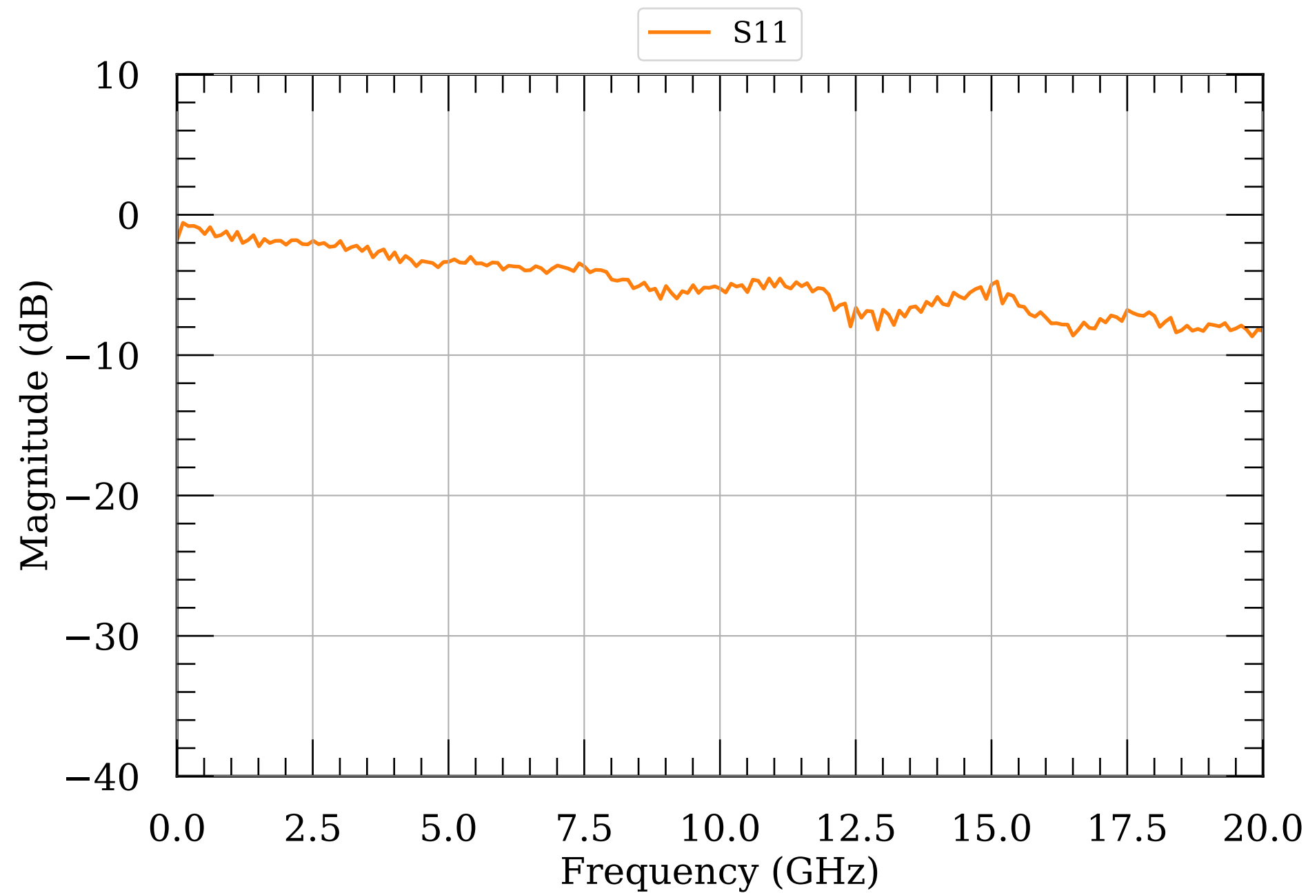
LNA S-params module005
